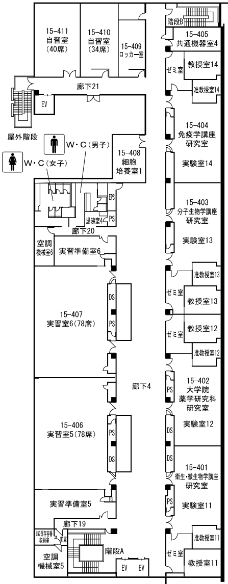
4階
