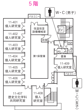
4階
